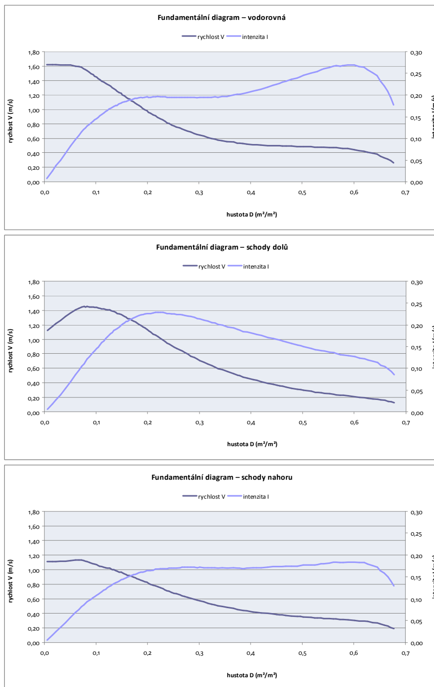
Obrázek 9.2: Fundamentální diagramy modelu
