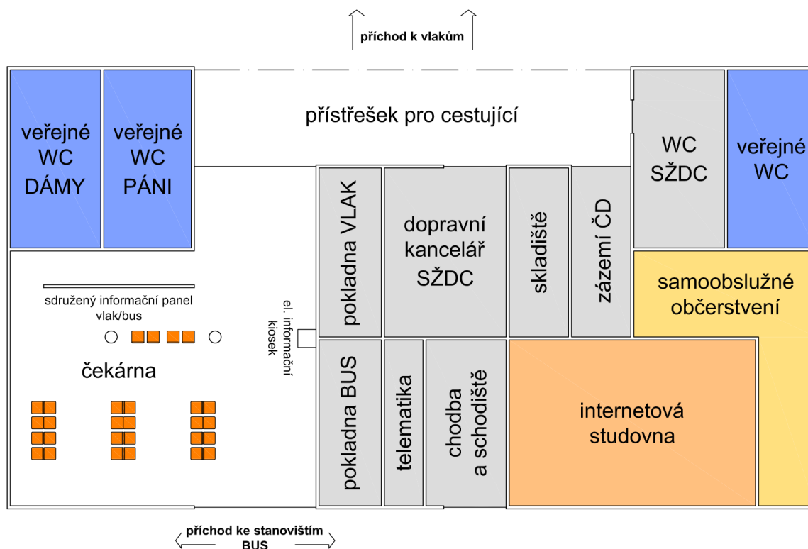
Obrázek 1.2: Žst. Vlašim – dispoziční řešení výpravní budovy
