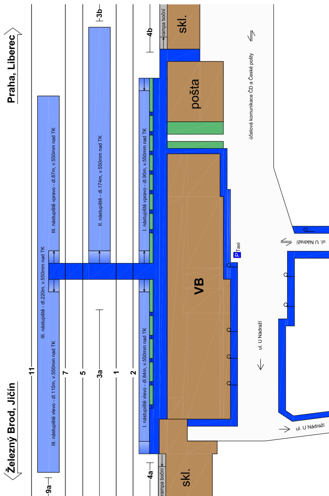
Obrázek 2.1: Turnov – příklad uspořádání přestupního uzlu veřejné hromadné dopravy
