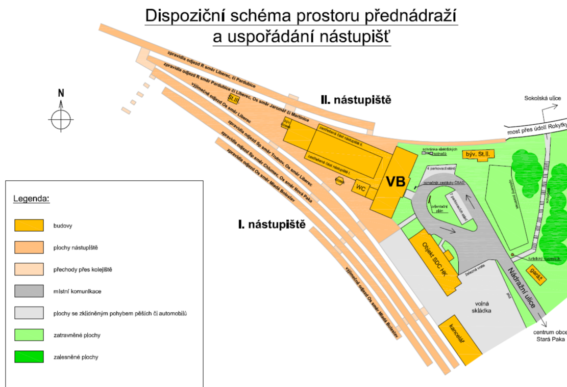
Obrázek 2.2: Stará Paka – příklad uspořádání přestupního uzlu veřejné hromadné dopravy
