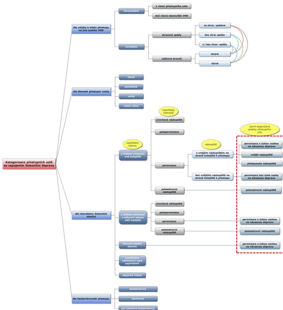
Obrázek 3.4: Kategorizační strom
